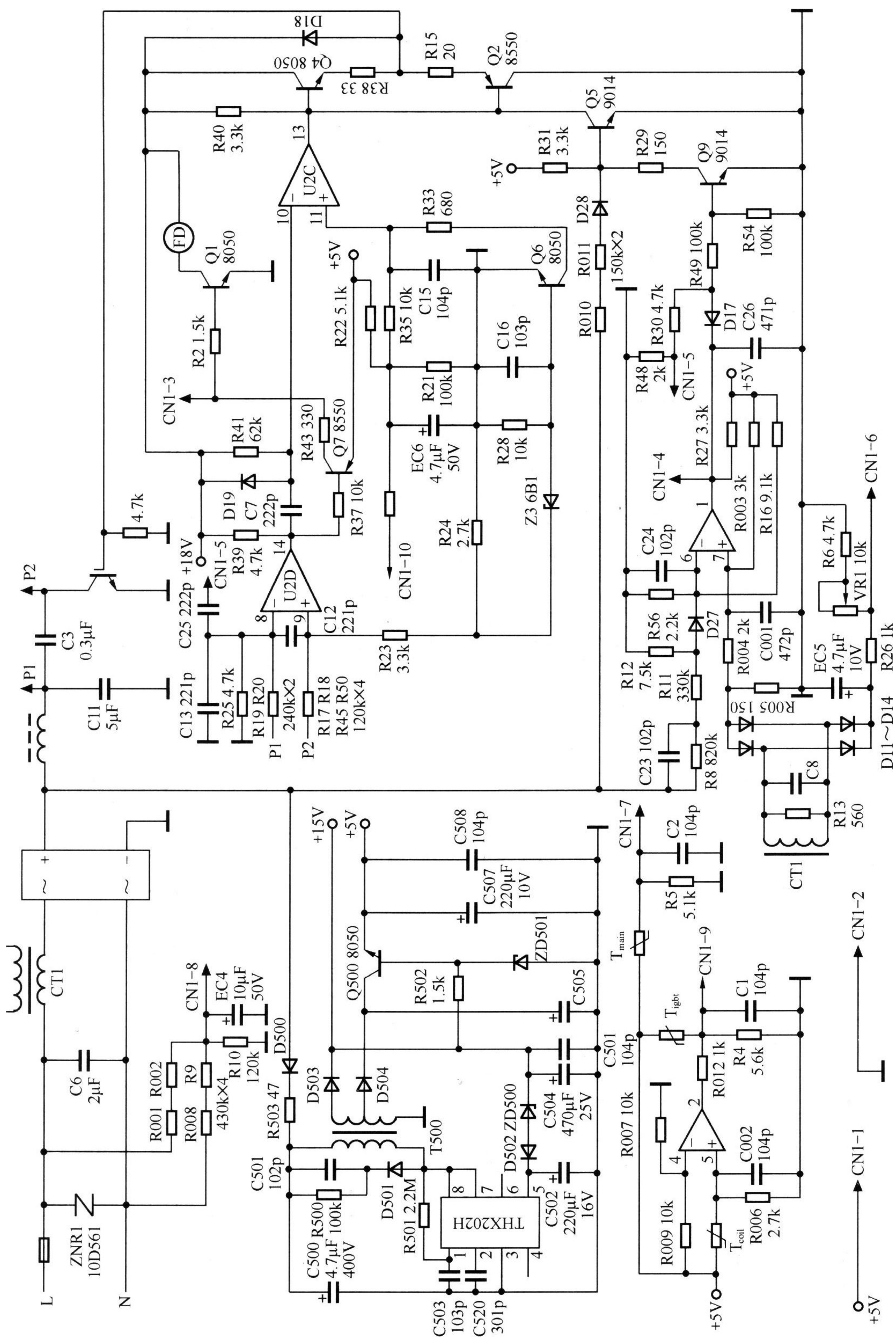
九阳 JYC-19POWER电磁炉主板电路原理图
